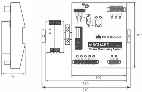
VIB7.900-PS ICPシステムモジュール寸法
