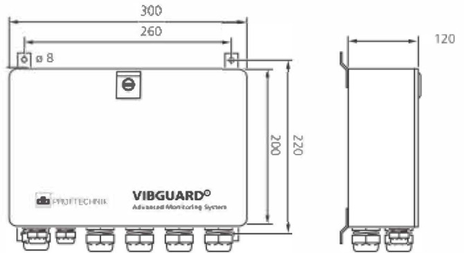
VIB7.900-LHハウジング寸法
